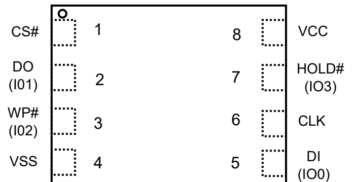
WSON 6x5 / USON 2x3
